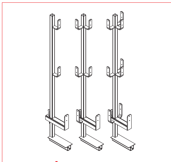
Słupki - trzy rodzaje
