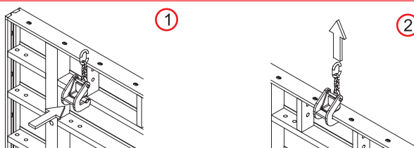
Zawiesie transportowe - przykład montażu
