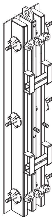
Element rozszalowujący
