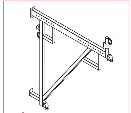
Wspornik szalunku wspinającego
