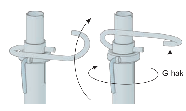
Kolejność postępowania przy odciążaniu podpory przy użyciu G-haka
